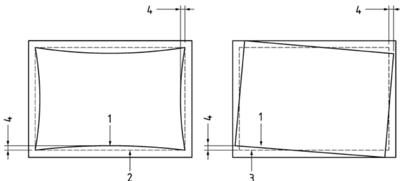
Bild F.2 — Beispiele für Abweichungen des Abstandhalters
